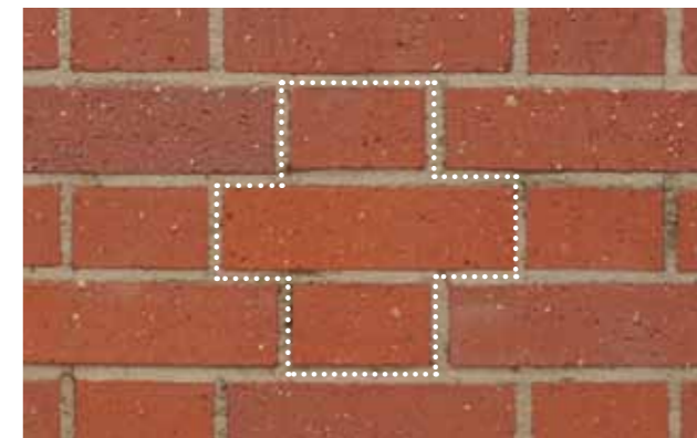
Die Hervorhebung in diesem Bild zeigt den Kreuzverband.
